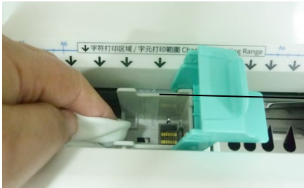
Держатель картриджа печати
